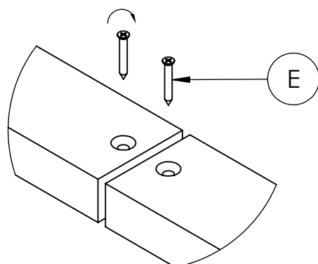
Detalj E 1:2
