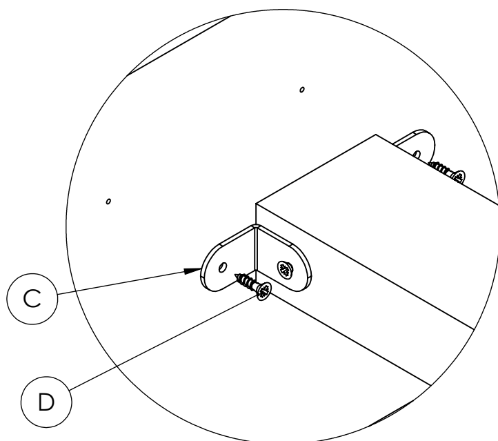
Detalj C 1:2
