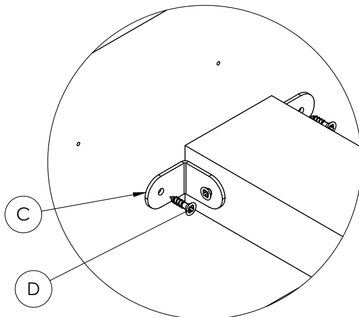
Detalj C 1:2
